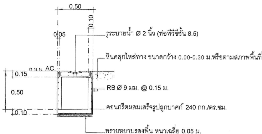
รูปตัด A-A รางระบายนํ้า
