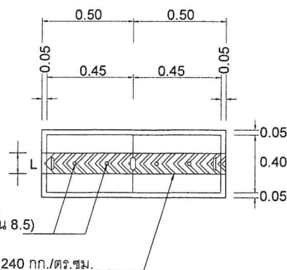
แบบขยายฝารางระบายนํ้า
