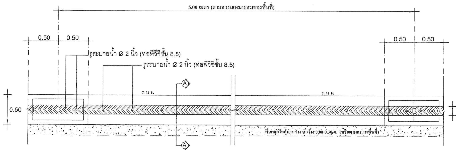
แปลนรางระบายนํ้า คสล.(แบบขยาย 1)
