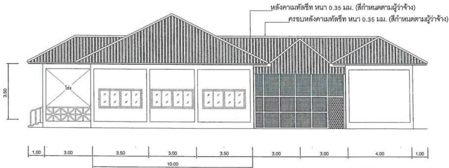
รูปด้าน 2
