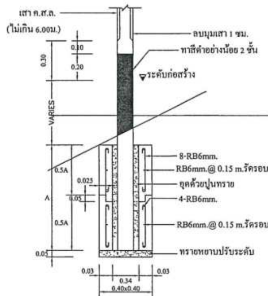
ขยายฐานเสา
