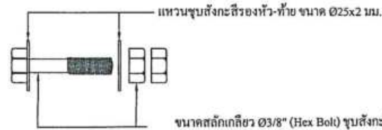
ขยายสลักเกลียว
